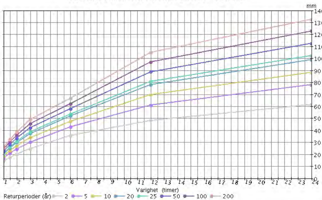
Figur 3.11: IVF-kurver (i millimeter) for 50480 Bergen-Sandsli (1982-2007) for 1-60 minutter (øverst) og 1 – 24 timer (nederst).
